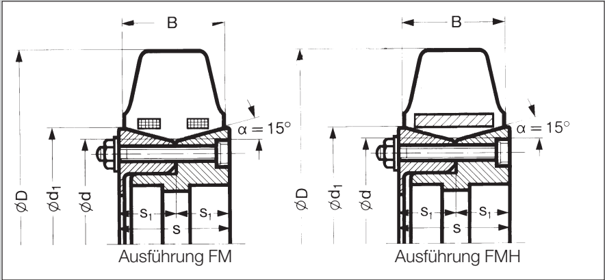
Abb. 5 ROTAFRIX® Führungsrollen mit Radkörpern
